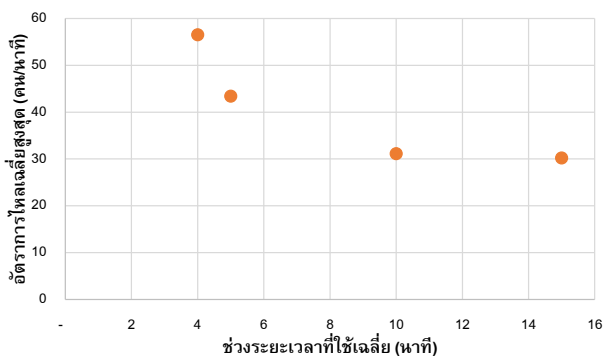
รูปที่ 8 แนวโน้มค่าอัตราการไหลเฉลี่ยต่อนาที่สูงสุดตามช่วงระยะเวลาที่เฉลี่ย
