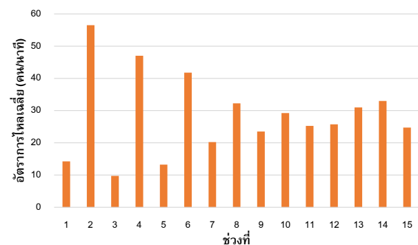
รูปที่ 4 อัตราการไหลเฉลี่ยต่อนาทีเมื่อใช้ช่วงระยะเวลาเฉลี่ย 4 นาที
